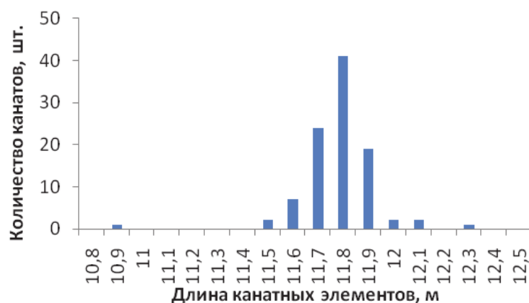
Рисунок 13 – Разброс длины канатных элементов гужевого пояса трала с фабричным размером 12,0 м
