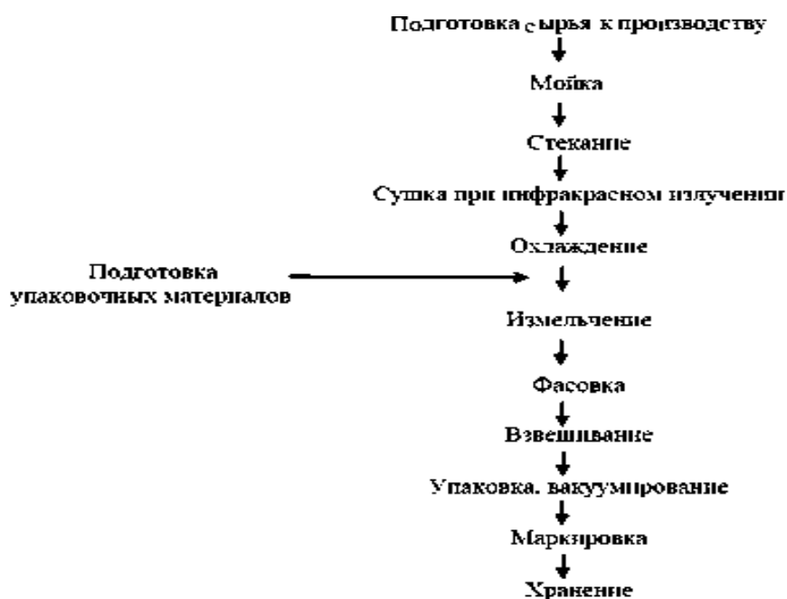
Рисунок 2 – Технологическая схема производства пищевого обогатителя из покровных тканей кальмара
