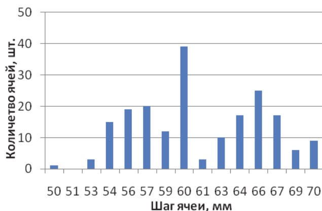
Рисунок 5 – Разброс размера ячеей сетной пластины с фабричным шагом 60 мм
