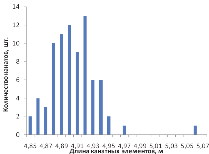
Рисунок 12 – Разброс длины канатных элементов трала с фабричным размером 5,0 м
