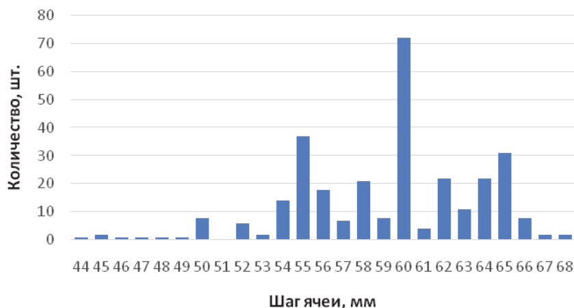
Рисунок 4 – Разброс размеров ячеей селективной вставки, перпендикулярных оси трала
