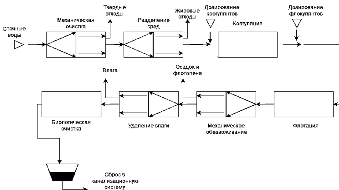
Рисунок 2 – Операторная модель очистки сточных технологических вод на АО «Южморрыбфлот»
